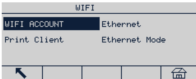
Figura 3-85: Opzioni WiFi
