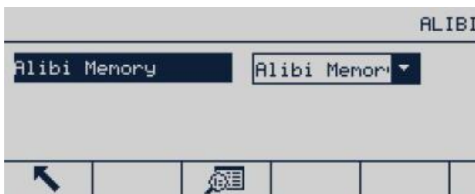
Figura 3-39: Menu Alibi
