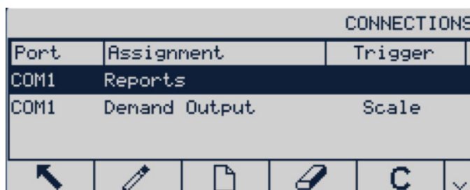
Figura 3-53: Elenco collegamenti
