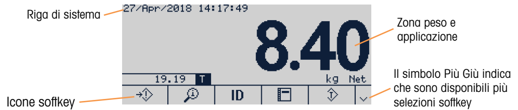
Figura 2-8: Display principale
