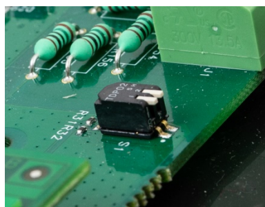
S1-1 spento
