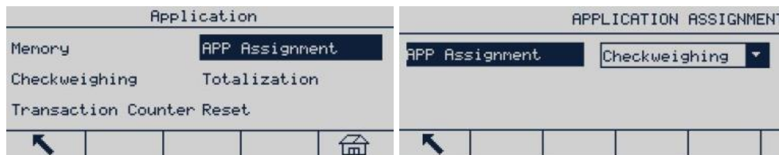
Figura 3-56: Configurazione applicazione
