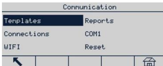
Figura 3-74: Menu comunicazione
