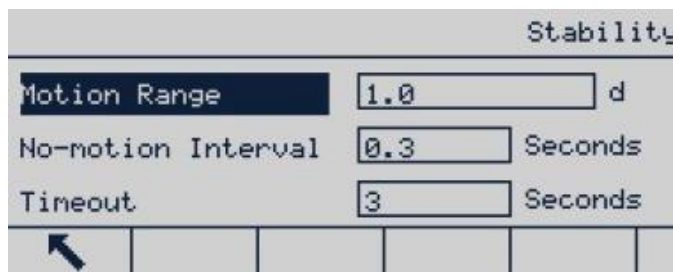
Figura 3-34: Schermata stabilità
