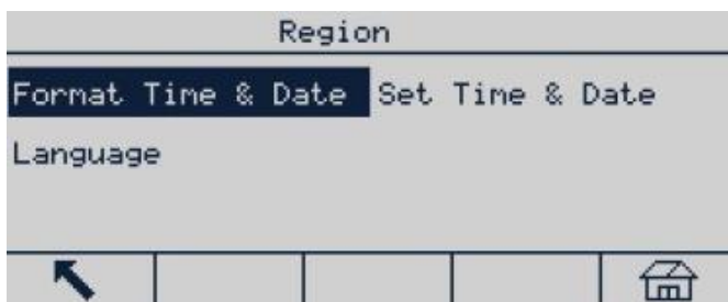
Figura 3-67: Menu Paese/nazione
