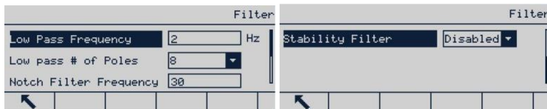
Figura 3-33: Schermate filtro
